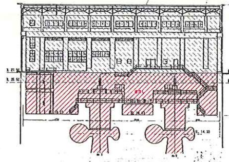
発電所側面図
